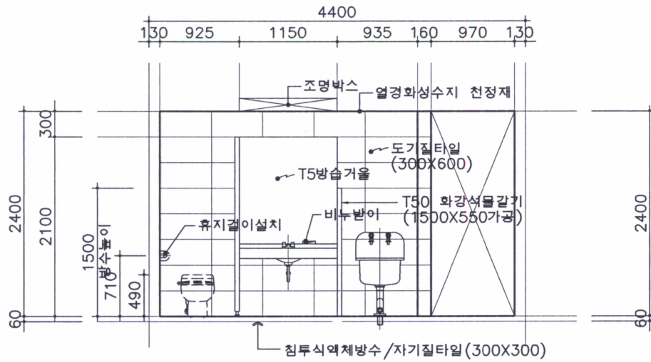
"C" 전 개 도
