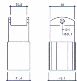
받침대 상세도 SCALE : 1/3
