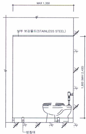
칸막이입면도(일반)-2 축척 : 1/30
