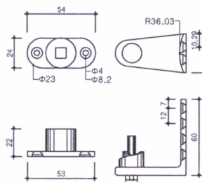
하부 피벗힌지 SCALE : 1/3
