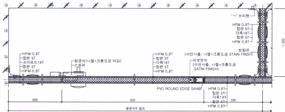
평면도 축척 : 1/30
