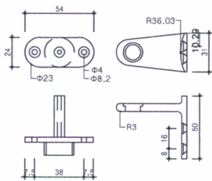
상부 피벗힌지 SCALE : 1/3
