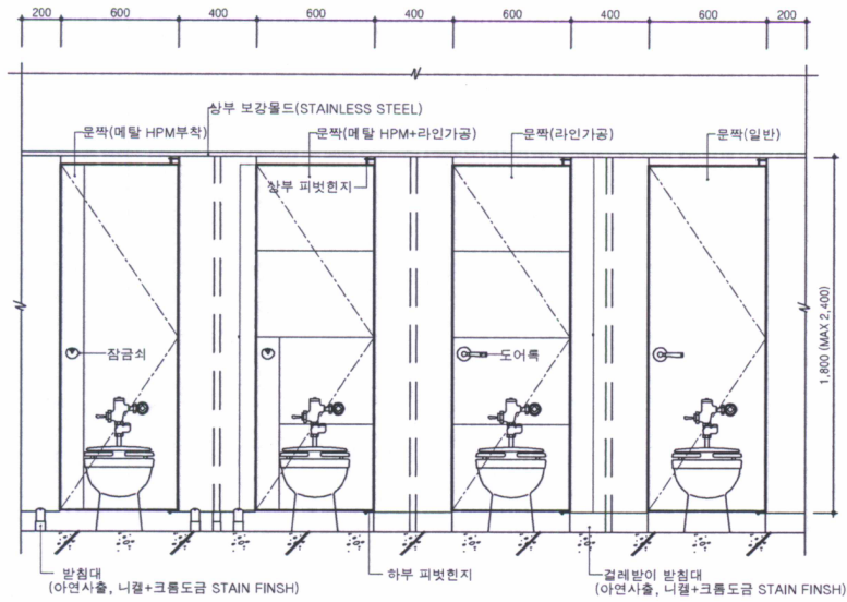
칸막이입면도(일반)-1 축척 : 1/30
