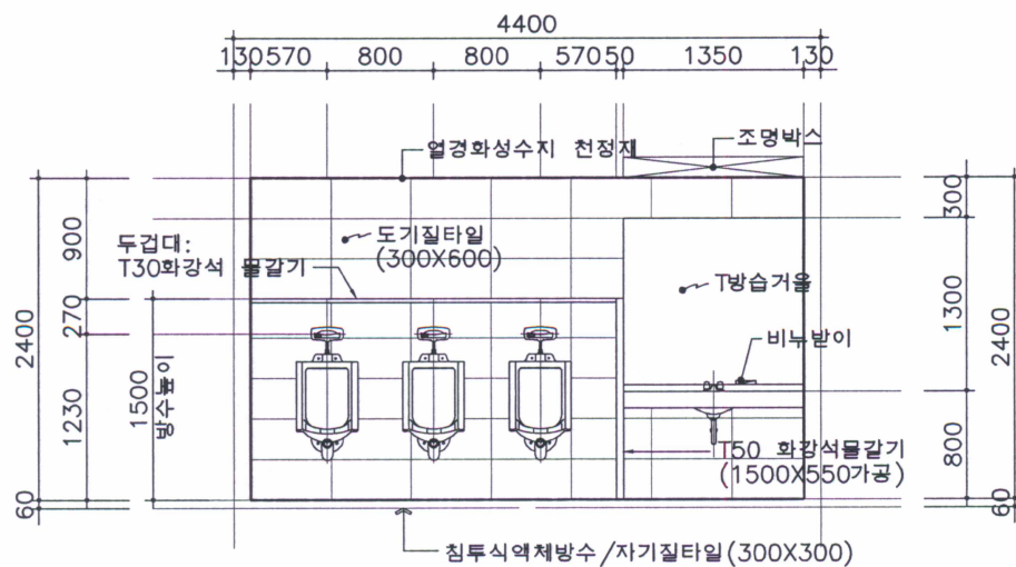
"E" 전 개 도
