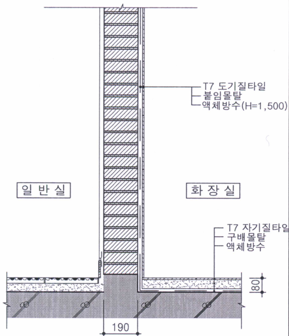
1 화장실 방수 상세도
