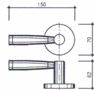
도어 록 SCALE : 1/5
