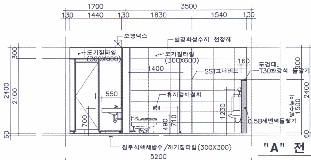
화장실평면상세
