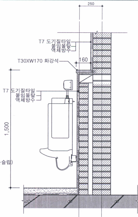
2 화장실 상부벽 상세도
