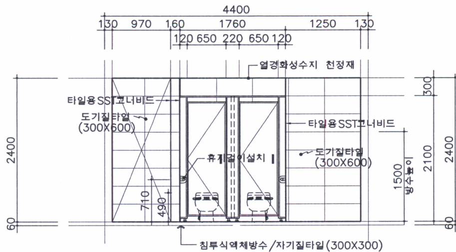
"D" 전 개 도
