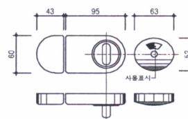
잠금쇠 SCALE : 1/5
