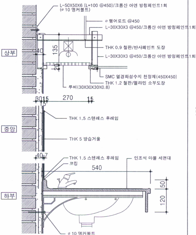
3 세면기 단면(조명박스)상세도
